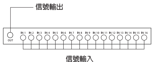
(2) 數位電視十六路混合主機 (機櫃式) MIXD-16C
