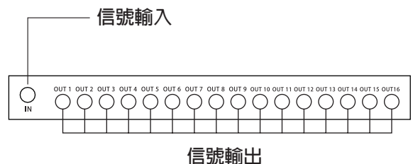
(2) 衛星電視十六路分配主機 (機櫃式) SPBS-16C
