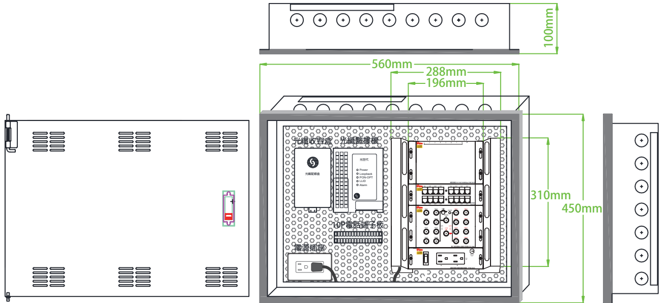
宅內弱電配線箱 尺寸：450(H)×560(W)×100(D) mm
